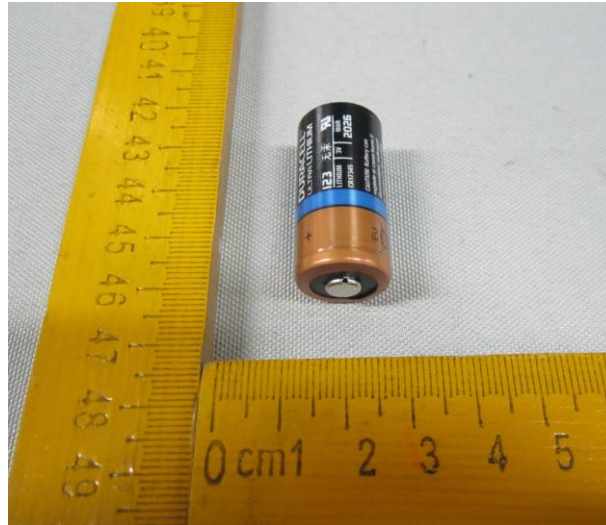
电池/ Battery(CR123 3V 1400mAh)
